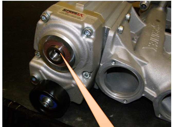
Seal journal
