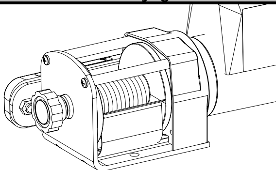
Embrayage
