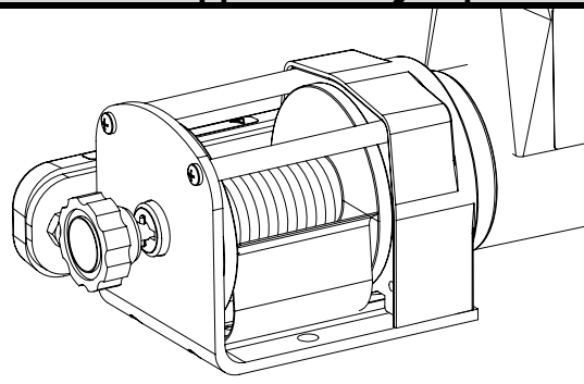
Ontkoppelen - vrijloop
